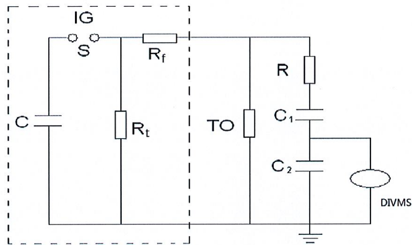
雷电冲击耐受电压试验回路图
