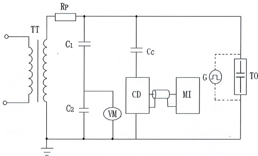
局部放电试验回路图
